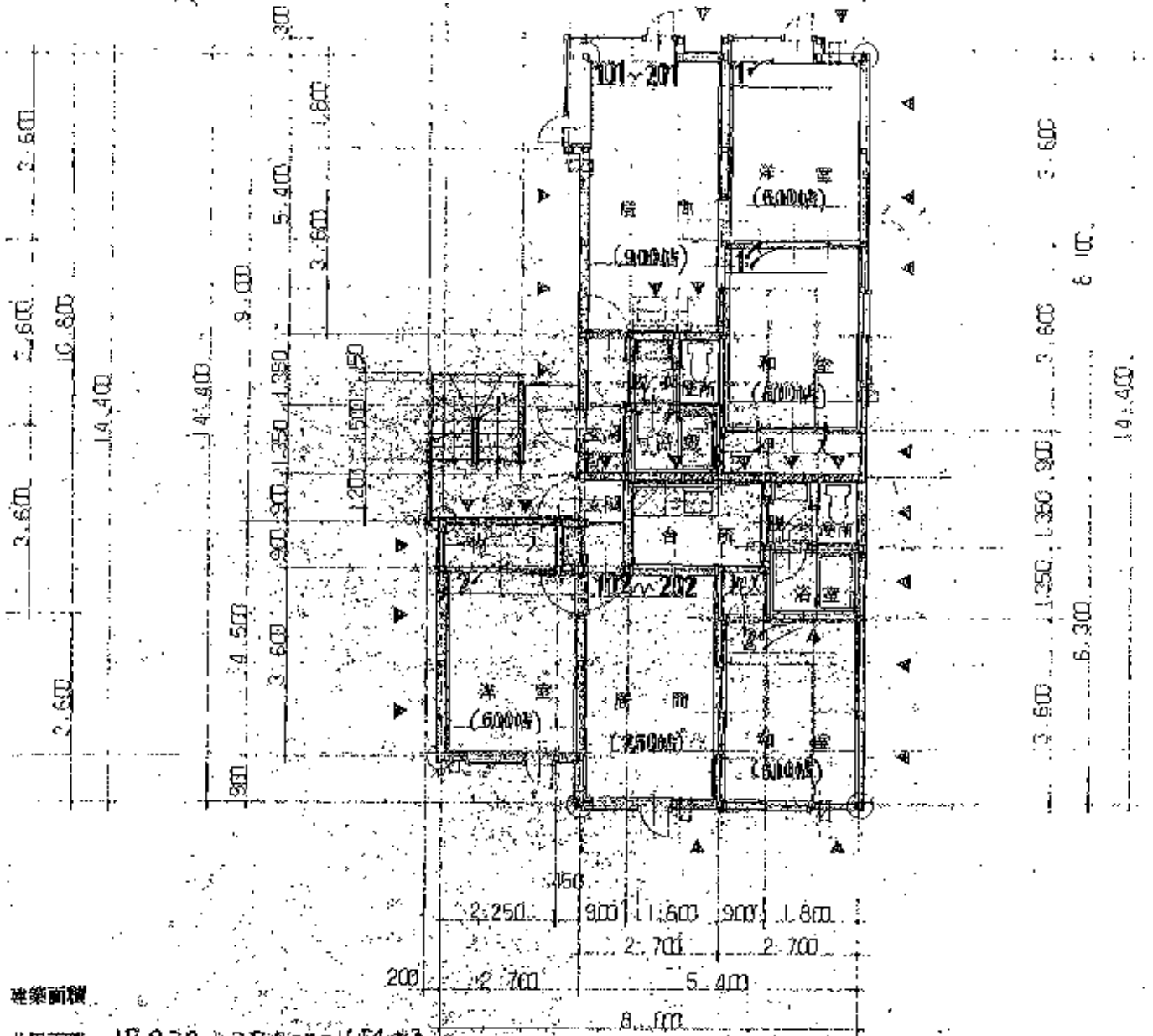
1、2階平面図 1:100
