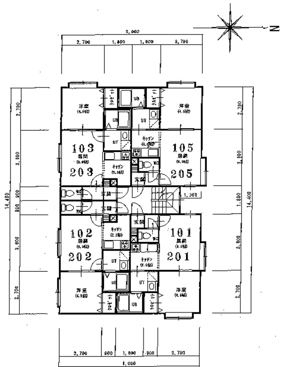
1F・2F平面図1/100
