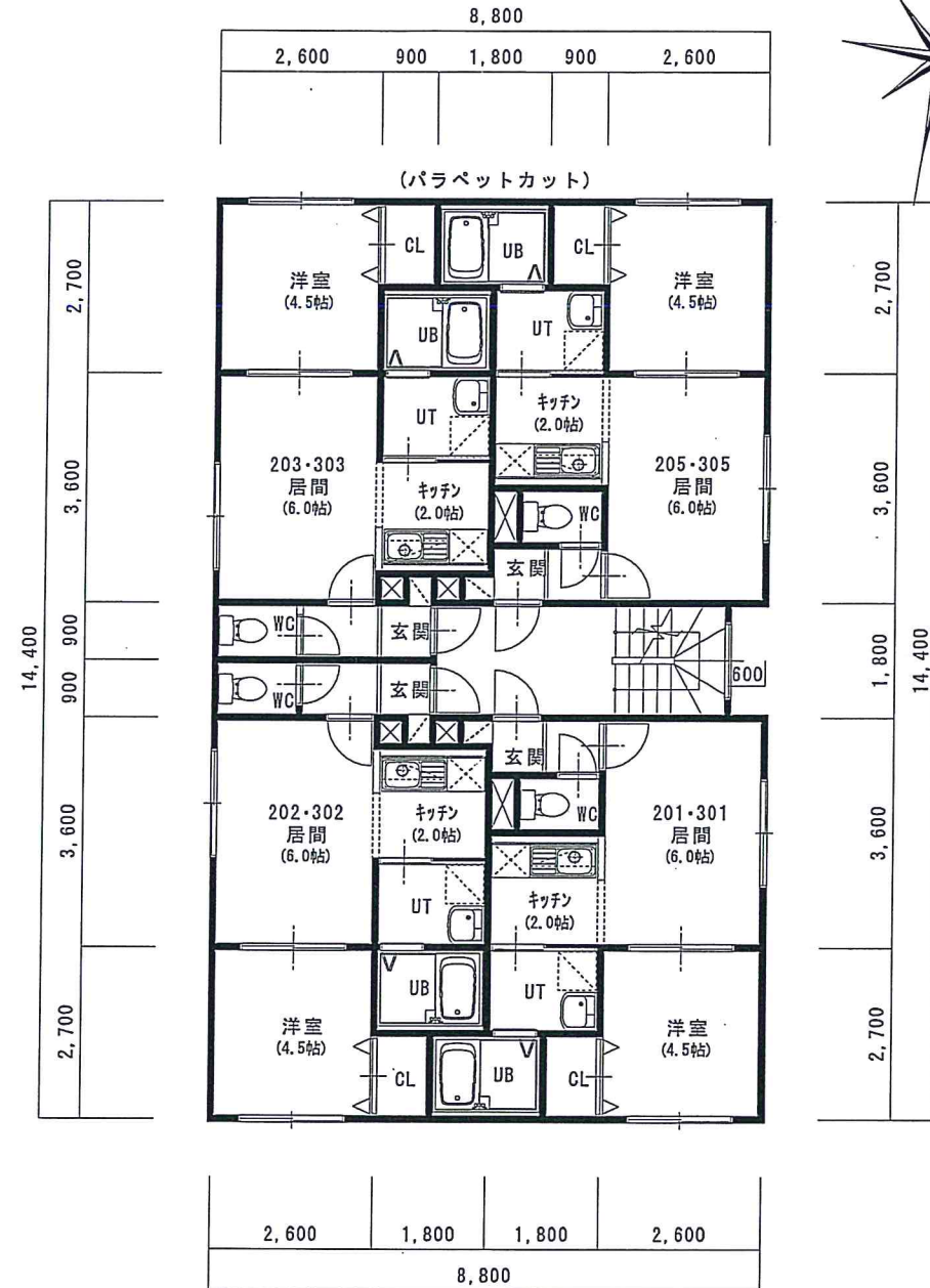
1F・2F平面図1/100
