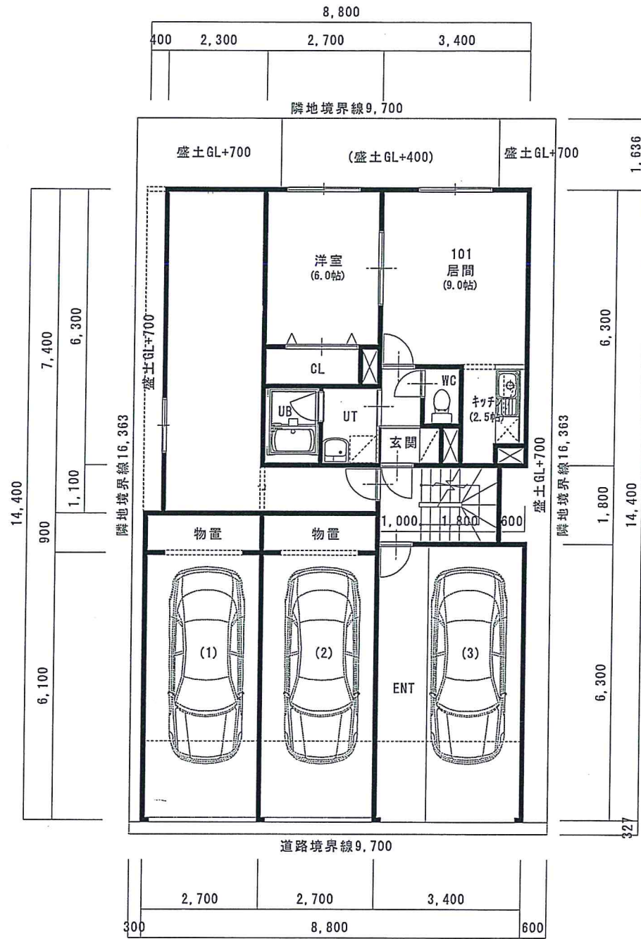
配置図・地階平面図1/100
