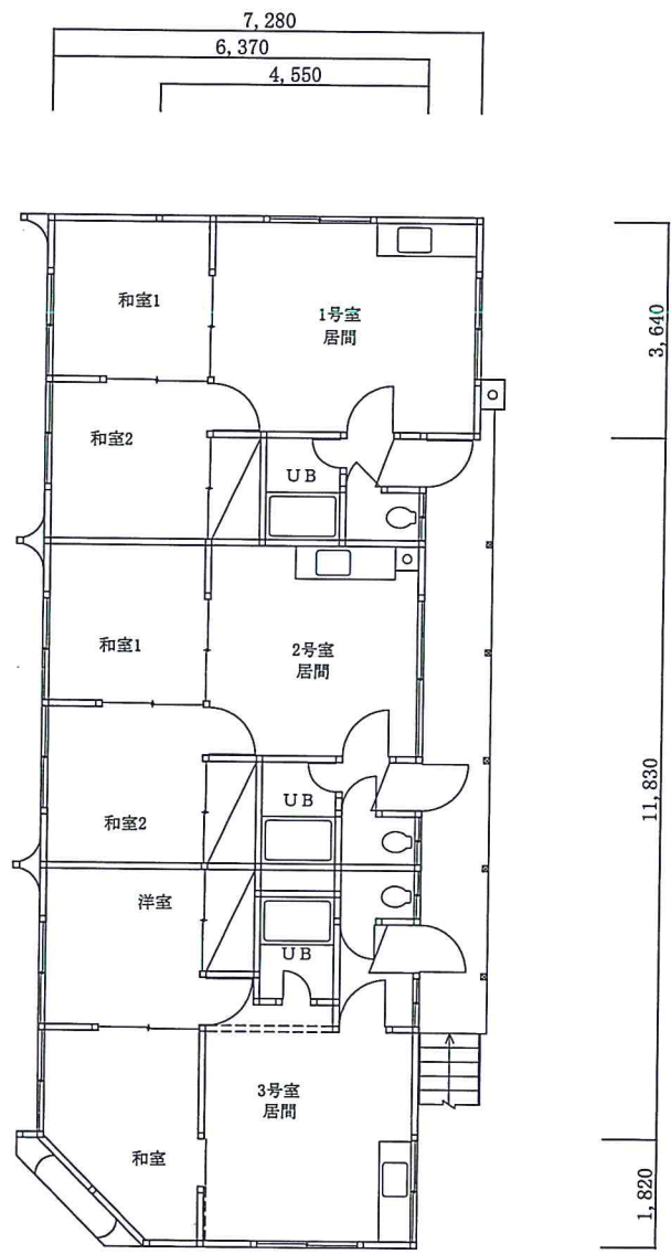
2階平面図
