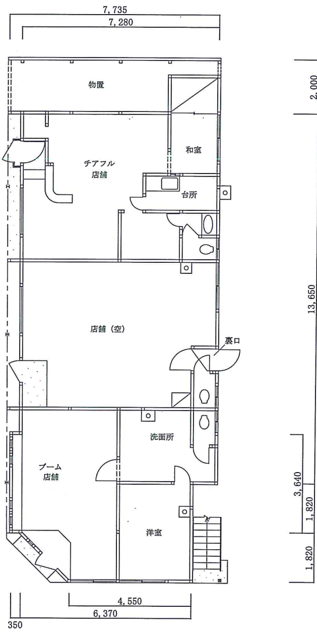
1階平面図
